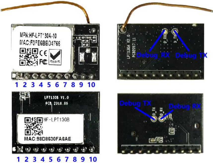
Figure 8. HF-LPT130A&B 管脚定义
