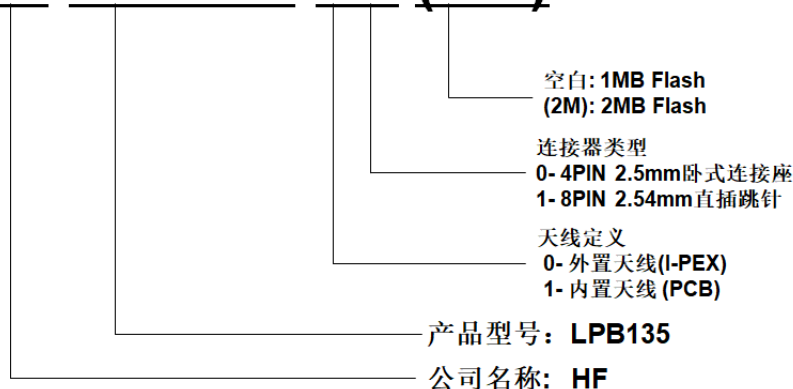
Figure 27. HF-LPB135 产品编号定义
