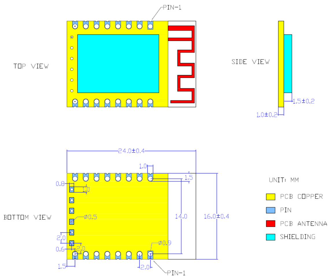
Figure 15. HF-LPT330 机械尺寸
