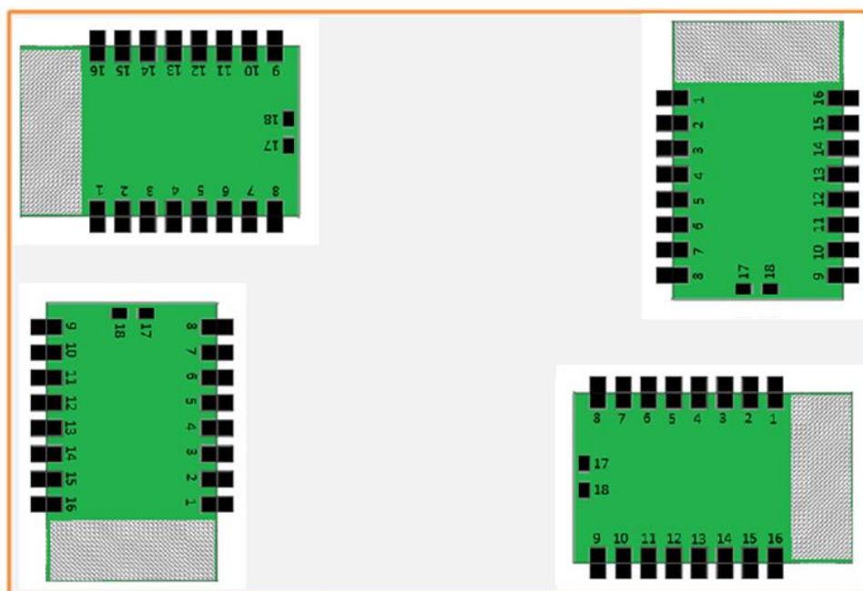
Figure 18. HF-LPT230 模组建议放置区域
