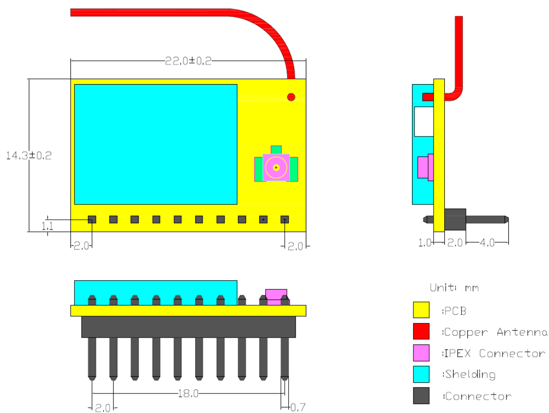
Figure 13. HF-LPT130A 机械尺寸
