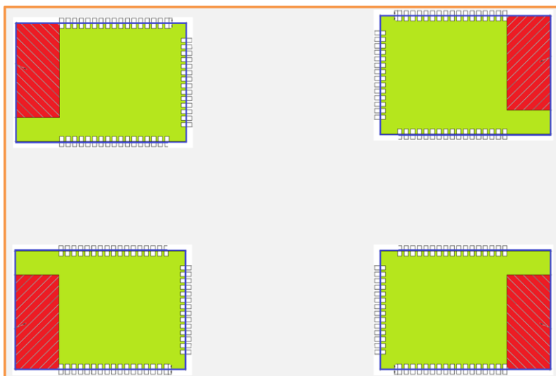
Figure 17. HF-LPB130 模组建议放置区域
