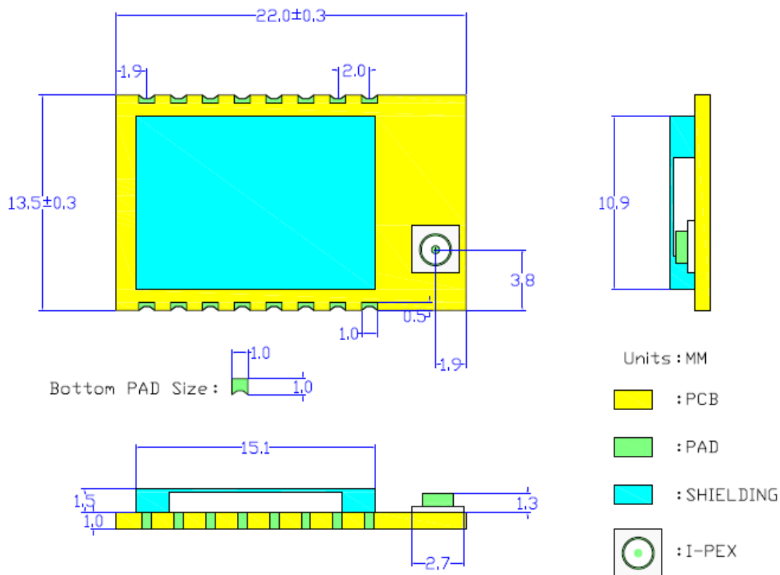
Figure 12. HF-LPT230 机械尺寸
