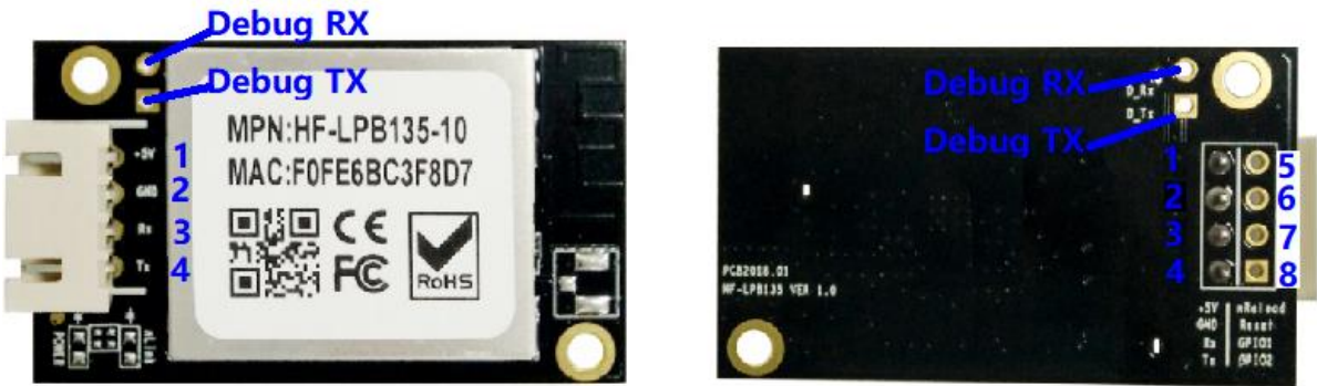
Figure 10. HF-LPB135 管脚定义
