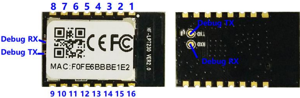
Figure 7. HF-LPT230 管脚定义
