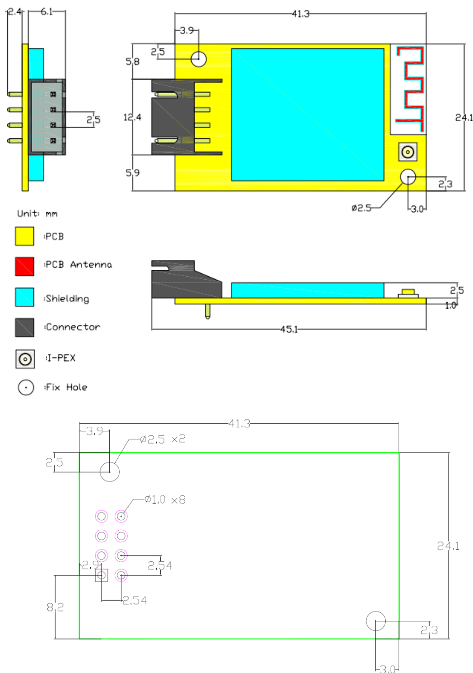
Figure 16. HF-LPB135 机械尺寸
