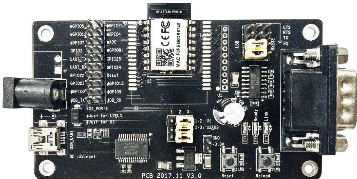
Figure 21. HF-LPT230 开发板
