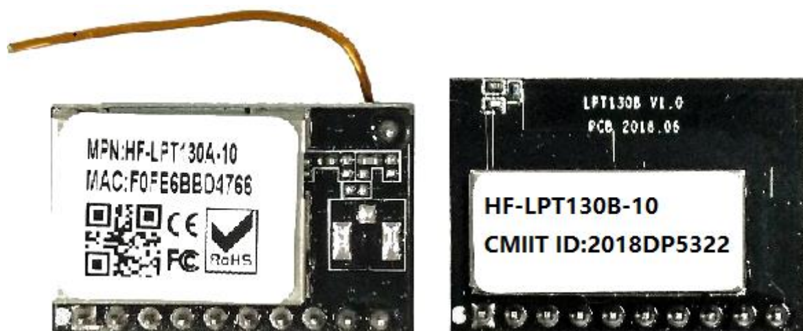
Figure 3. HF-LPT130A-10 和 HF-LPT130B-10 外观图
