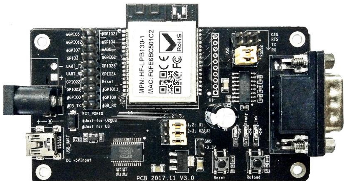
Figure 20. HF-LPB130 开发板
